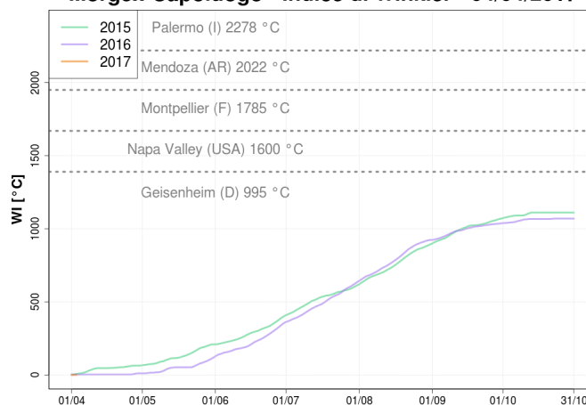
Morgex-Capoluogo - Indice di Winkler - 04/04/2017
