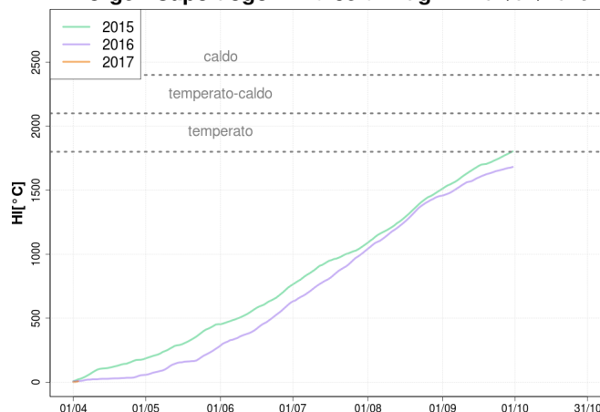
Morgex-Capoluogo - Indice di Huglin - 04/04/2017
